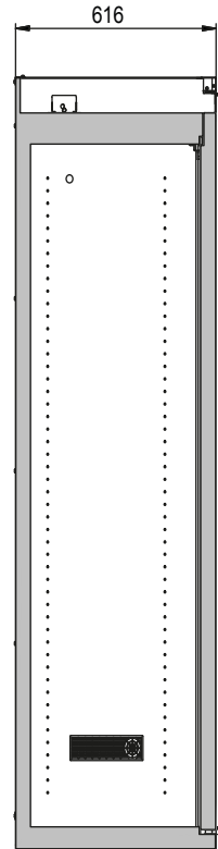
Vista lateral
